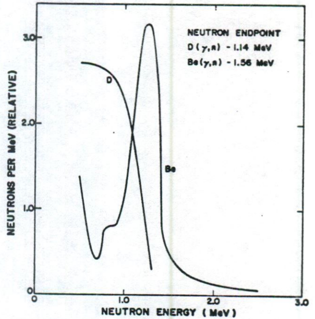
Fig. D-3. Deuterium and beryllium photoneutron spectra, 4.5-MeV bremsstrahlung.
